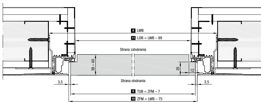
Horizontálny rez typu NA s normálnym otváraním krídla dverí
