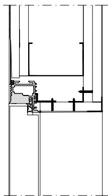
Vertikálny prierez normálne otváranie smerom von (typ NA)
