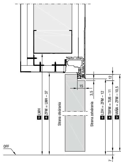
Vertikálny rez typu RI s reverzným otváraním krídla dverí
