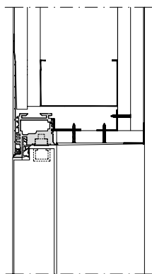
Vertikálny reverzný otvor do dverného otvoru (typ RI)
