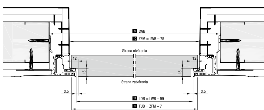
Horizontálny rez typ RI s reverzným otváraním krídla dverí
