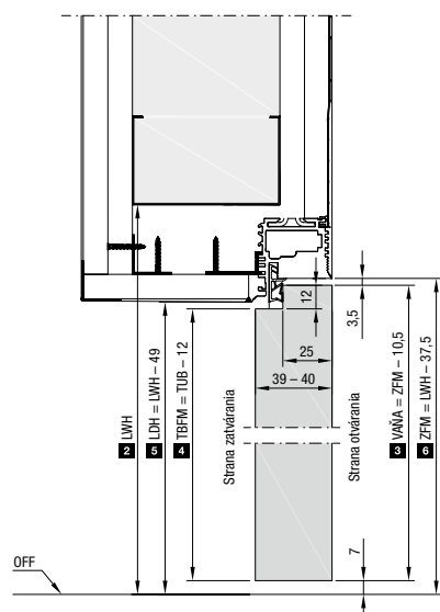
Vertikálny rez typu NA s normálnym otváraním krídla dverí
